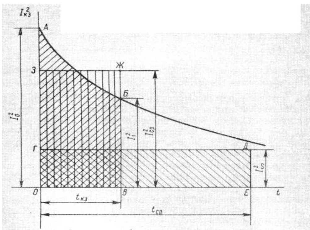
Рисунок 3 - График для определения фиктивного времени КЗ
